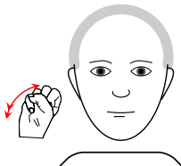
b. KIMATI+++
