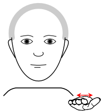
(1) a. OTROK
