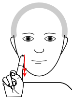
(2) a. MAMA
