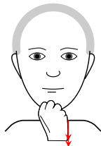
(3) a. JABOLKO
