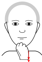
b. JABOLKO
