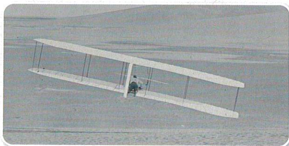
Wilbur Right leta 1902 med treningom zavijanja z jadralskim letalom
