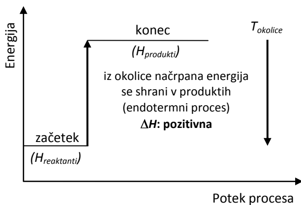
Shema 2: Energjski diagram endotermnega procesa
