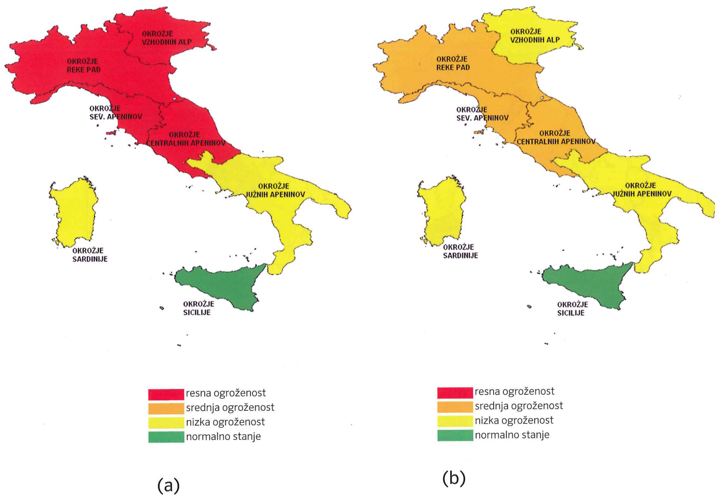
Slika 6: Intenziteta suše na državni ravni: (a) stanje avgusta 2022; (b) stanje decembra 2022
