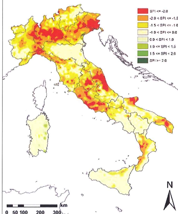
Standardizirani padavinski indeks (SPI) za obdobje mar-apr-maj 2022
