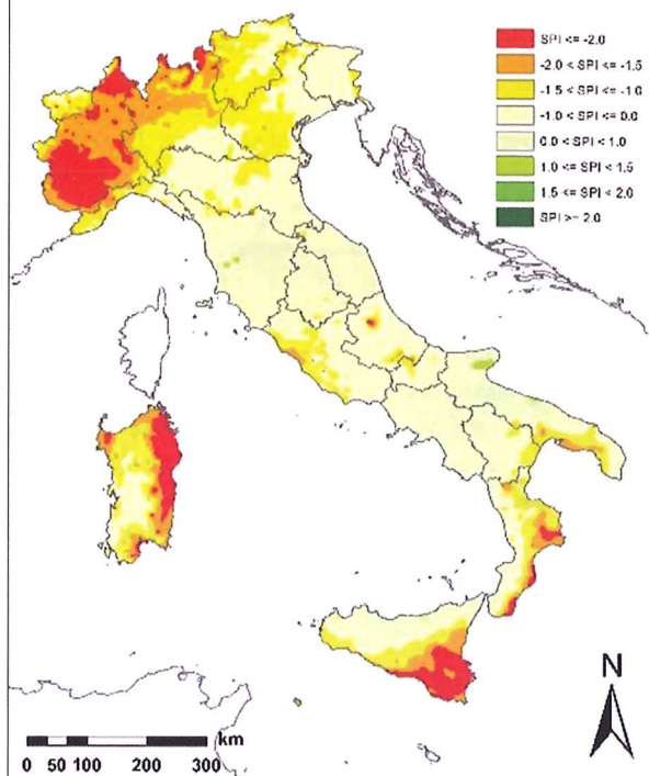
Standardizirani padavinski indeks (SPI) za obdobje dec-jan-feb 2022
