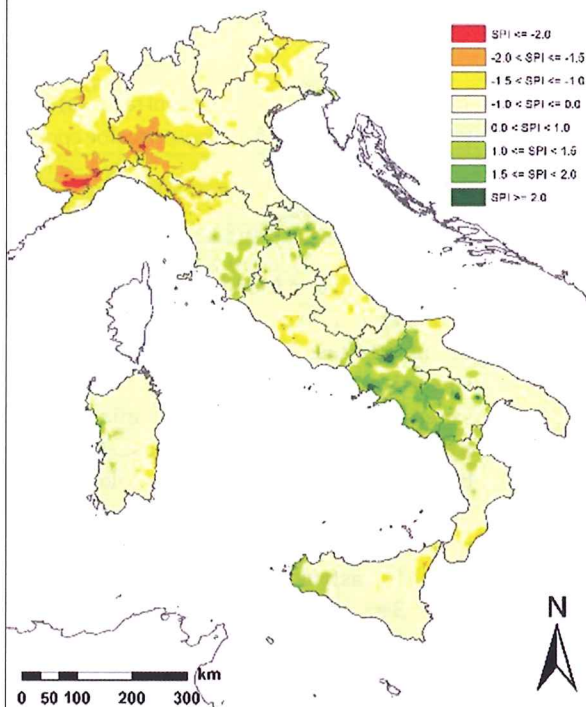
Standardizirani padavinski indeks (SPI) za obdobje sep-okt-nov 2022
