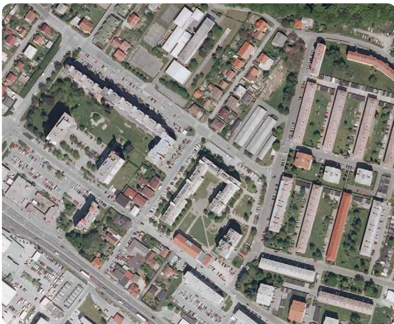
Del Maribora na letalski fotografiji
