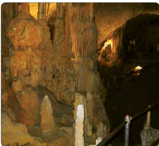
Slika 51: Postojnska jama
