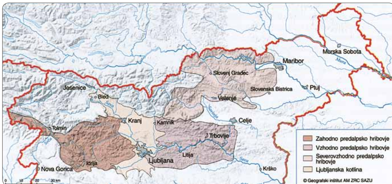
Slika 41: Polhograjsko hribovje
