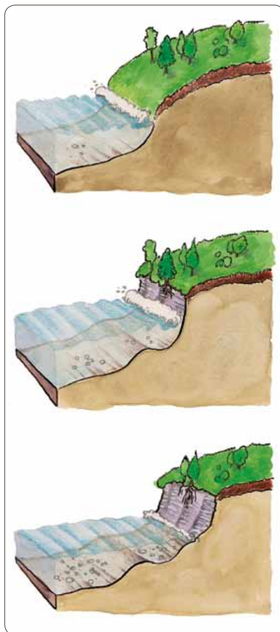
Slika 78: Nastajanje klifa
