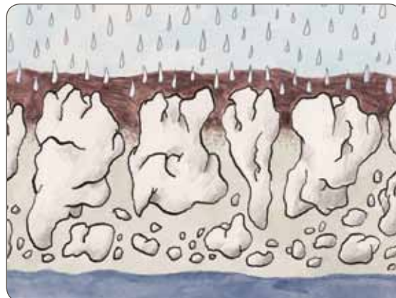
Slika 59: Delovanje vode na apnenec
