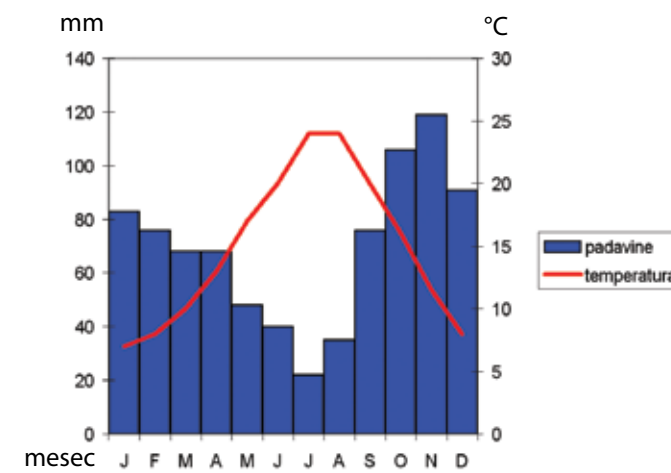
Klimogram za Rim
