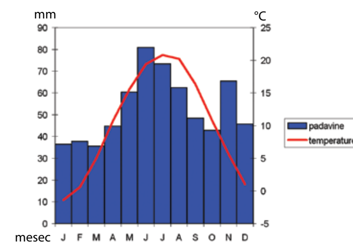
Klimogram mesta Siofok ob Blatnem jezeru na Madžarskem
