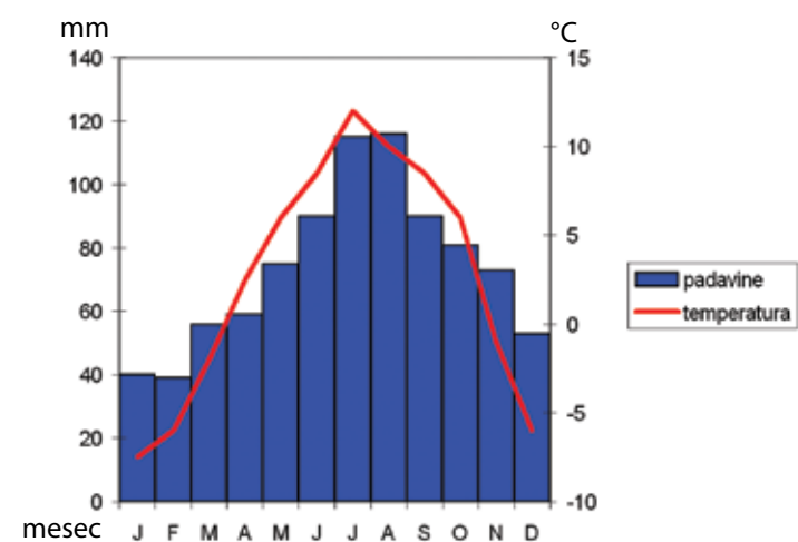
Klimogram švicarskega smučarskega središča St. Moritz
