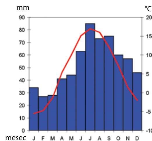
Slika 126: Klimogram za Rigo
