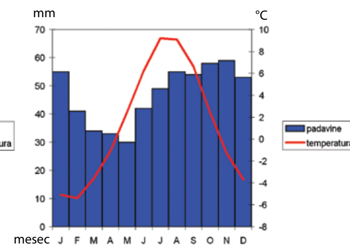
Slika 127: Klimogram za Vardo
