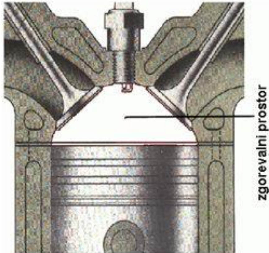
Slika 8: zaobljeni zgorevalni prostor
