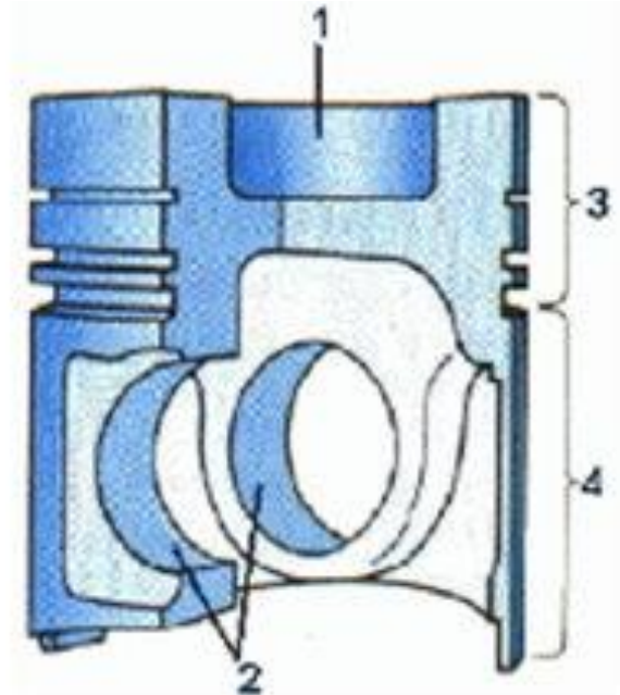
Slika 13: sestavni deli bata:
