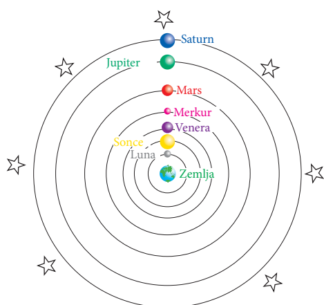
Aristotelov sistem
