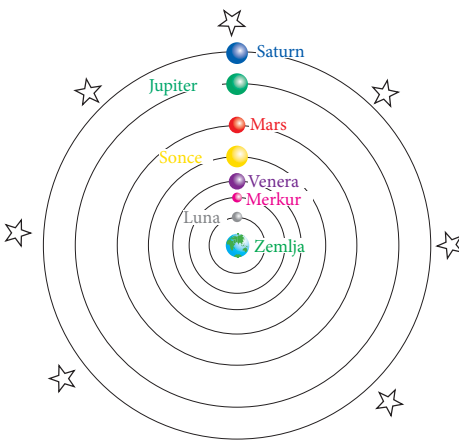
Ptolemejev sistem
