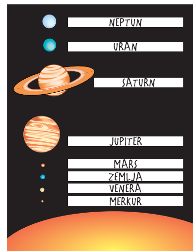
Današnji sistem
