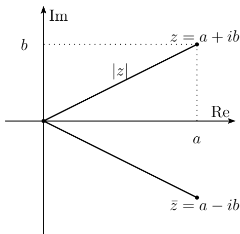
SLIKA 1.1. Realni in imaginarni del, absolutna vrednost in konjugirano število
