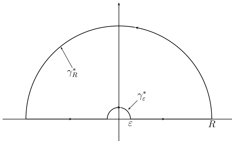
SLIKA 3.3. Integracijska krivulja \gamma
