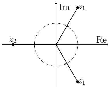
SLIKA 1.3. Rešitve enačbe z^3 = -1
